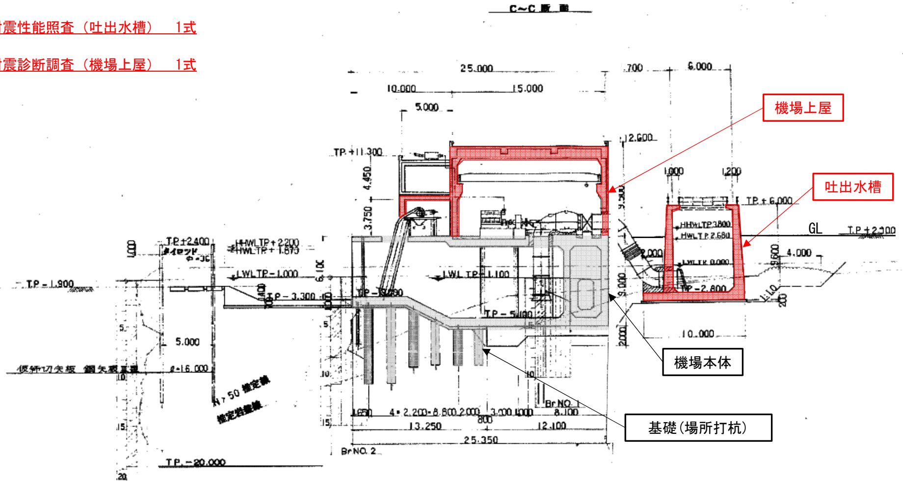
多々羅川排水機場 断面図(流水方向)
